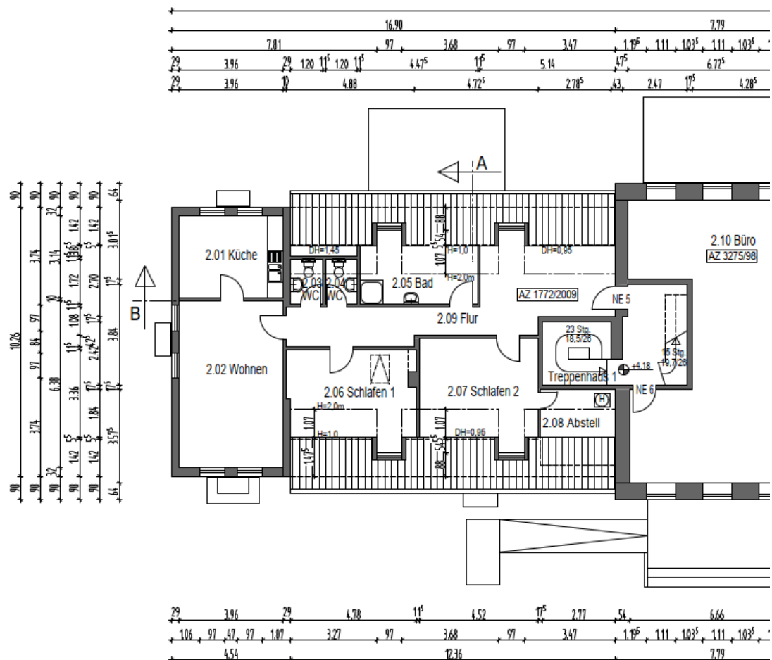
Grundriss Dach
